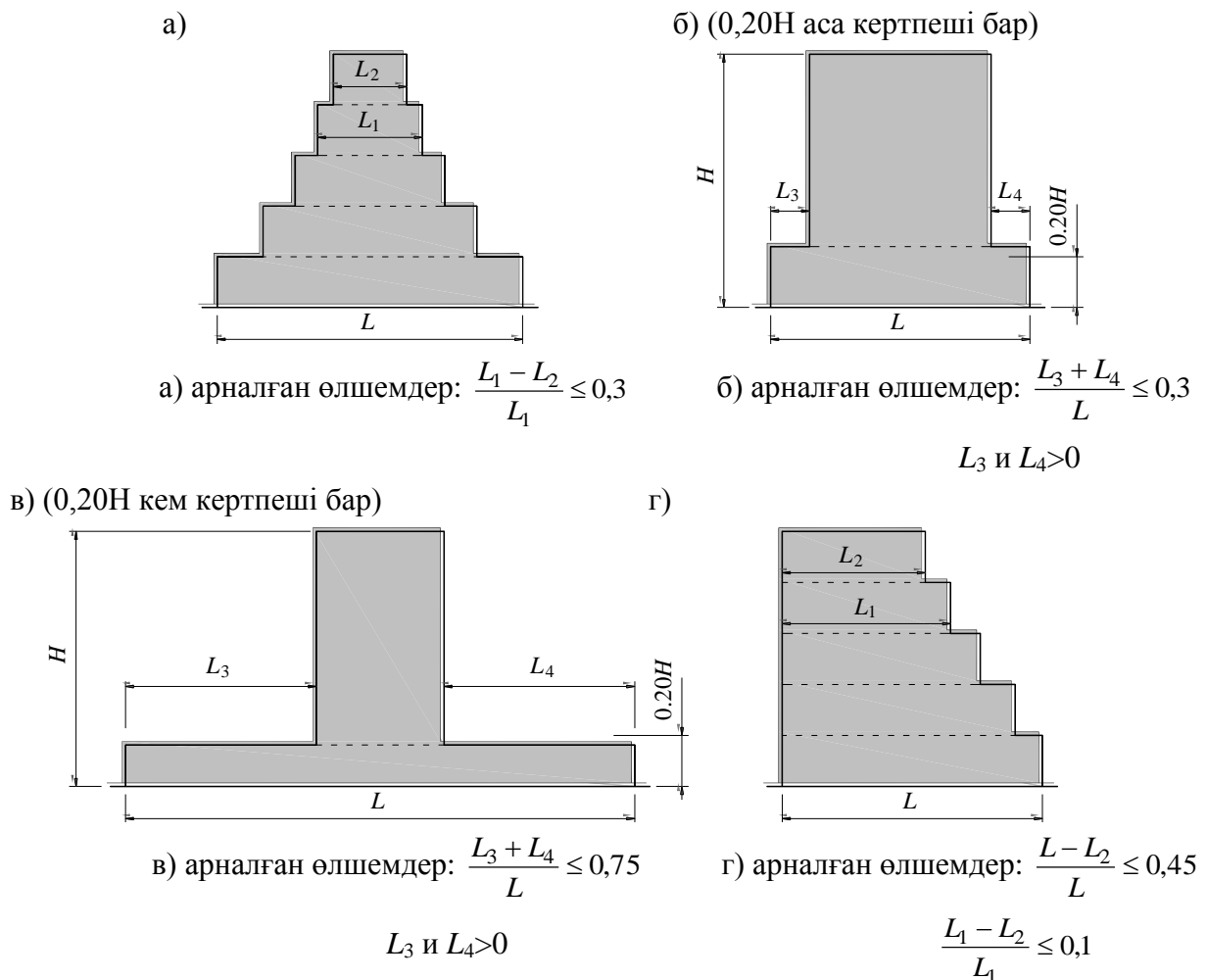
3.7-сурет – Кертпештері бар ғимараттарға арналған жүйелілік өлшемдері
