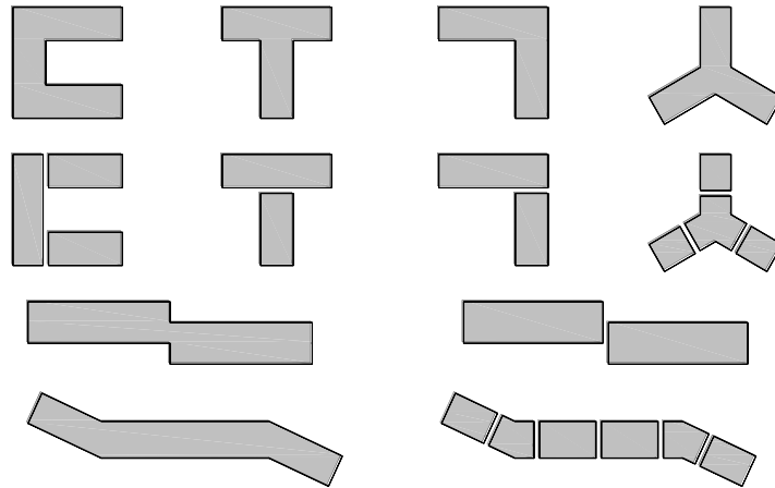
2.3-сурет – Жоспардағы күрделі формалары бар ғимараттардың динамикалық тәуелсіз бөлімшелерге бөлінуінің мысалдары
