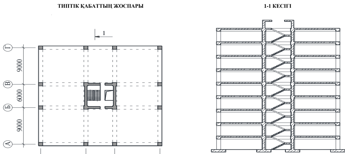
В.6-сурет – Қаңқаның схемалық жоспары, кесігі, жалпы түрі және есептік схемасы
