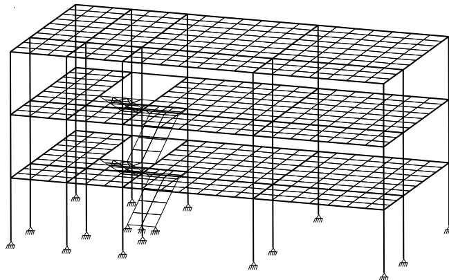
В.2-сурет – Ғимараттың есептік схемасы
