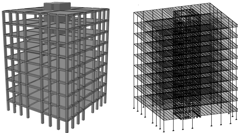
Рисунок В.9 – Общий вид и расчетная схема конструктивной системы
