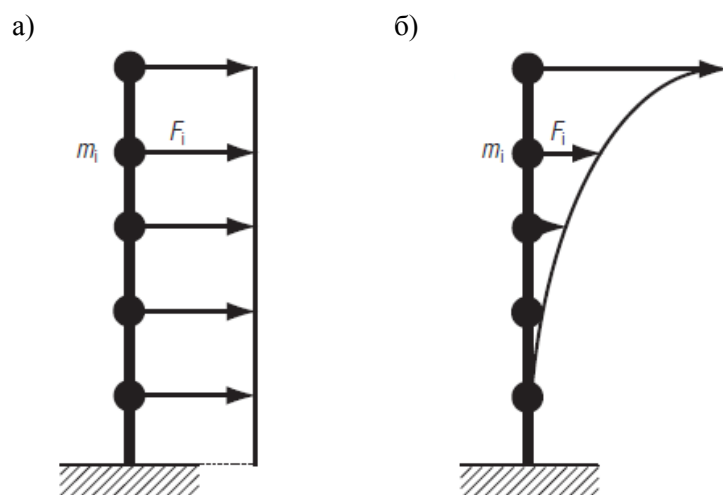
Б.1-сурет – Ғимараттың биіктігі бойынша қолбеу жүктемелерді орналастырудың екі схемасы
