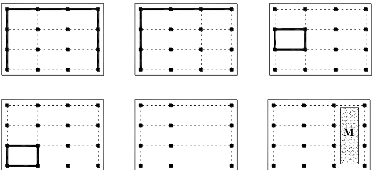
2.8-сурет – Жоспарда қаттылықты және/немесе массаларды (М) жүйесіз және үйлесімсіз бөлуі бар конструктивтік жүйелердің мысалдары
