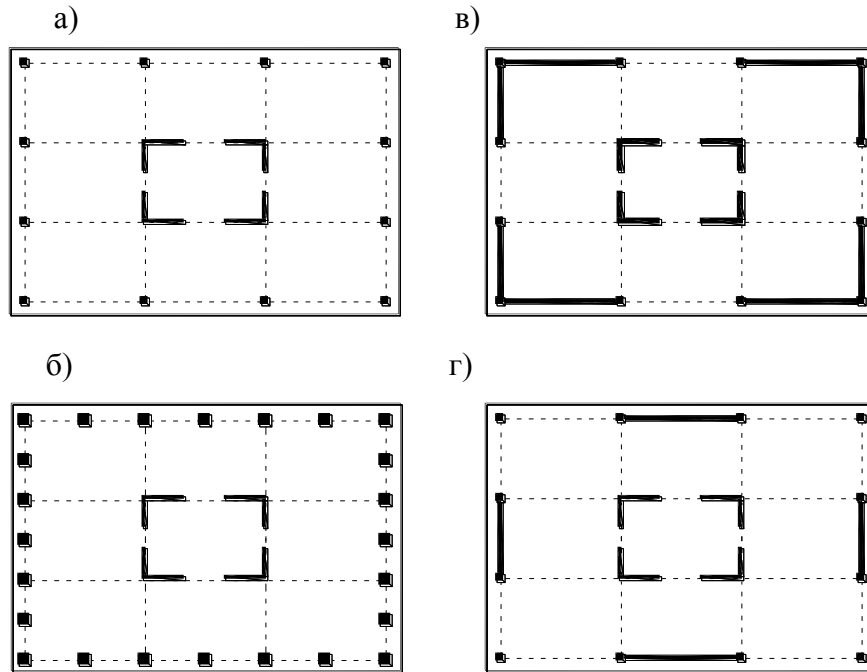
2.7-сурет – Жоспарда бұраудың а) төменгі және б), в), г) жоғары қарсылықтығы бар жоспардағы жүйелі және симметриялық конструктивтік жүйелердің мысалдары
