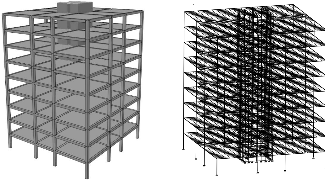
В.7-сурет – Қаңқаның жалпы түрі және есептік схемасы
