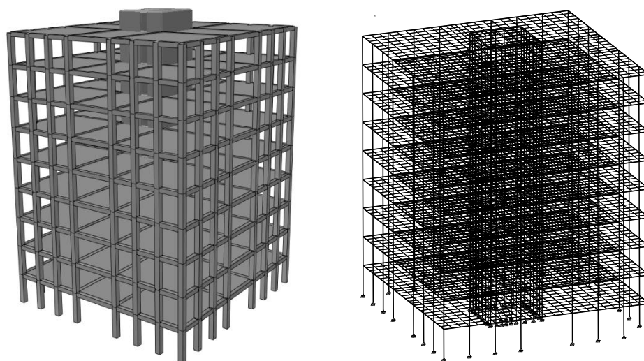
В.9-сурет – Қаңқаның схемалық жалпы түрі мен есептік схемасы
