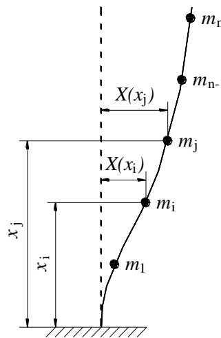
6.2-сурет – \eta_{ik} коэффициентінің мәндерін анықтау үшін
