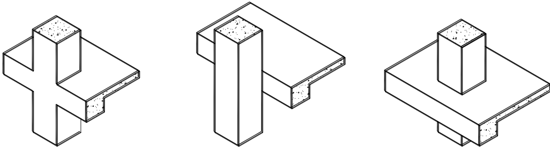
3.5-сурет – Беларқалардың бағандармен қосылудың эксорталықтың тораптардың мысалдары
