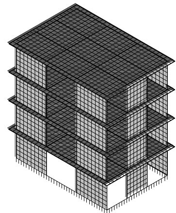
6.1-сурет – Ғимараттың жазық және кеңістіктің есептік модельдері
