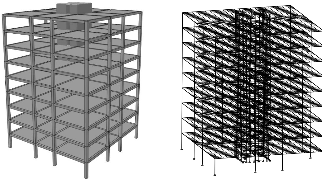
Рисунок В.7 – Общий вид и расчетная схема конструктивной системы
