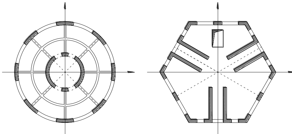
2.5-сурет – Жоспарда дөңгелек және дұрыс алты бұрышты түрдің формасындағы басты ортогоналдық бағыттарда жақын қаттылық пен қарсылықтығы бар конструктивтік жүйелердің мысалдары
