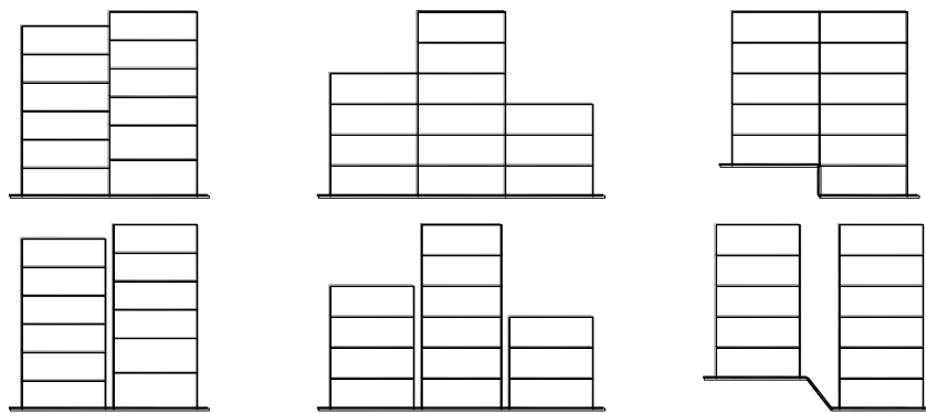
2.4-сурет – Биіктік бойынша күрделі формалары бар ғимараттардың динамикалық тәуелсіз бөлімшелерге бөлінуінің мысалдары
