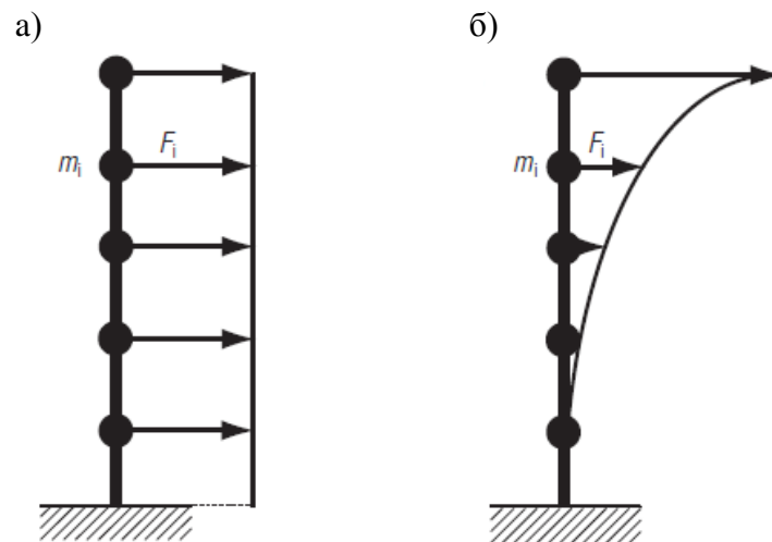
Рисунок Б.1 – Две схемы распределения горизонтальных нагрузок по высоте здания
