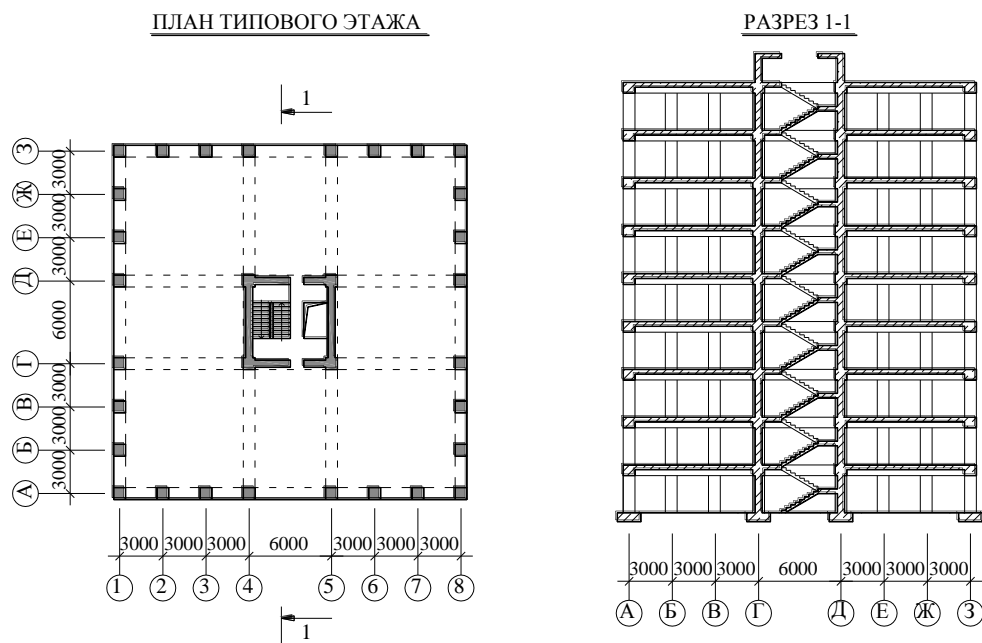
В.8-сурет – Қаңқаның схемалық жоспары мен кесігі
