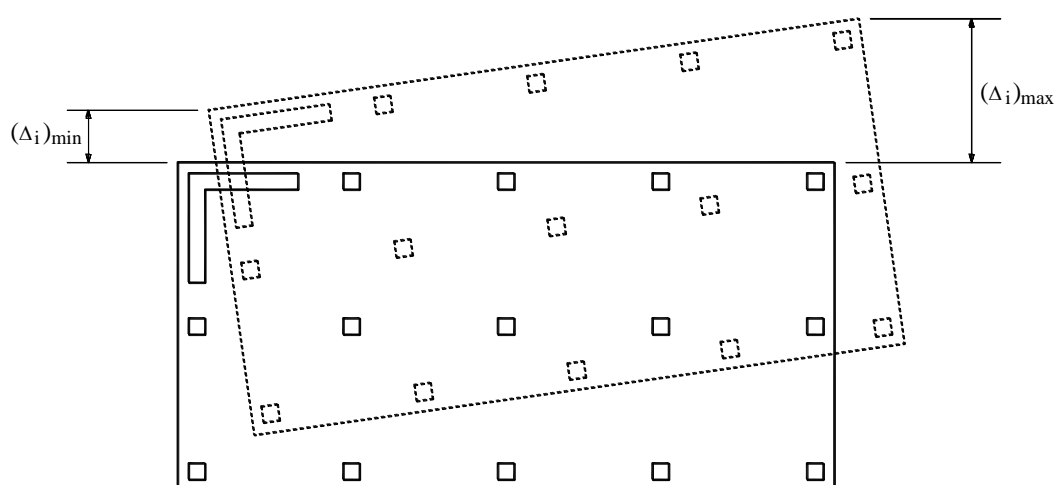
Рисунок 3.8 – К проверке горизонтальных перемещений в уровне перекрытий
