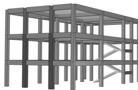
Рисунок В.4 – Схематический план и вид каркаса
