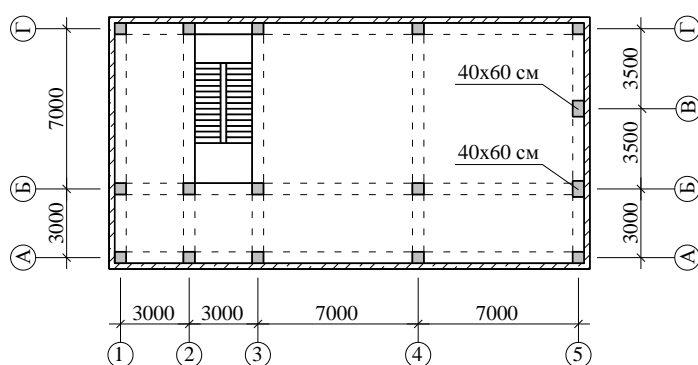
Рисунок В.4 – Схематический план и вид каркаса
