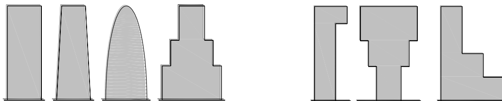
Рисунок 2.2 – Конфигурации зданий по высоте: а) благоприятные и б) неблагоприятные
