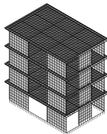
ПРОСТРАНСТВЕННАЯ РАСЧЁТНАЯ МОДЕЛЬ
