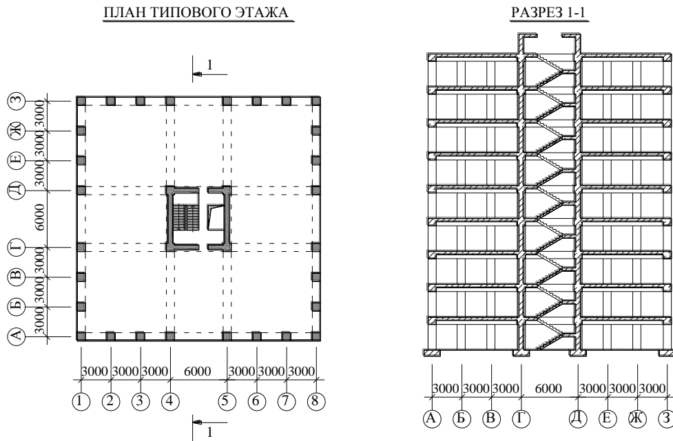
Рисунок В.8 – Схематические план и разрез
