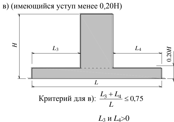
Рисунок 3.7 – Критерии регулярности для зданий с уступами
