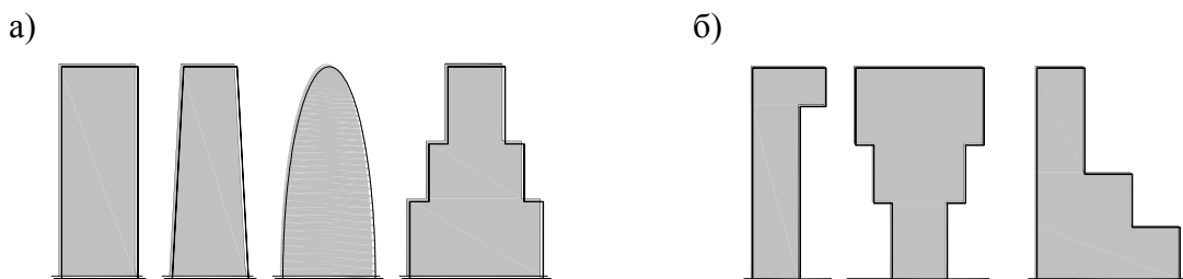
2.2-сурет – Ғимараттың биіктіктегі жағымды а) және жағымсыз б) конфигурациялары
