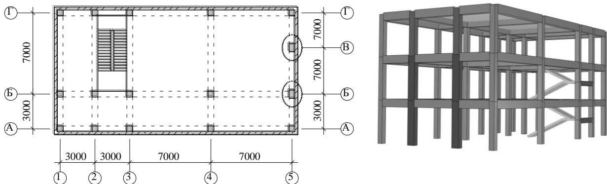
В.4-сурет – Қаңқаның схемалық жоспары мен түрі
