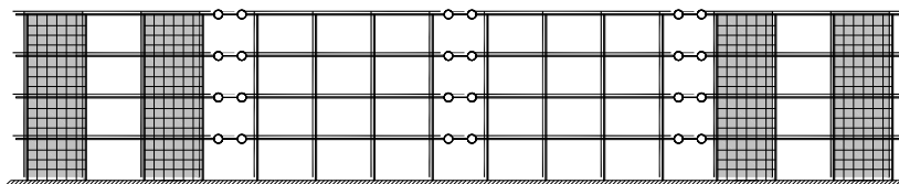
ПЛОСКАЯ РАСЧЁТНАЯ МОДЕЛЬ ПО ОСИ Y
