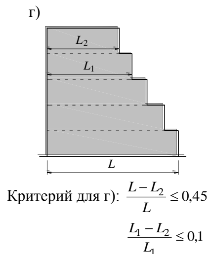
Рисунок 3.7 – Критерии регулярности для зданий с уступами
