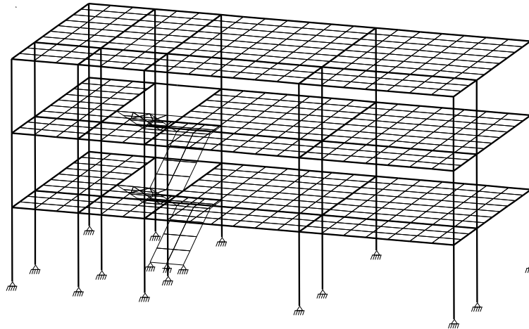
Рисунок В.2 – Расчетная схема здания
