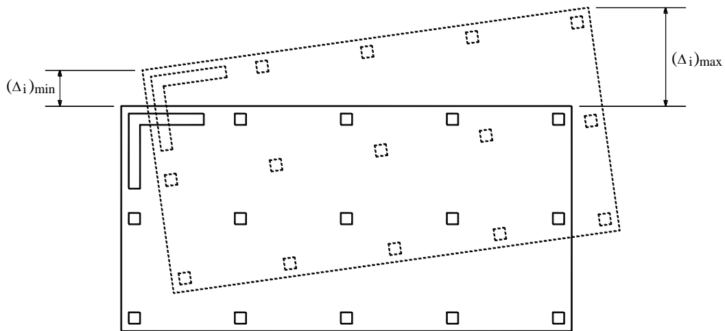
3.8-сурет – Арақабырға деңгейіндегі көлбеу орын ауыстыруларды тексеруге арналған
