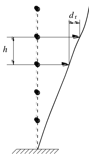
7.1-сурет – Қарастырылатын қабаттың жоғарғы және төменгі арақабырғаларының d_s орташа көлбеу орын ауыстыруларының d_r айырмашылығын анықтау үшін
