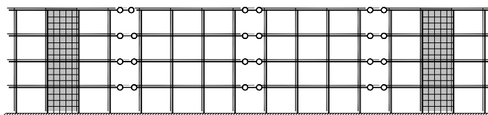
6.1-сурет – Ғимараттың жазық және кеңістіктің есептік модельдері
