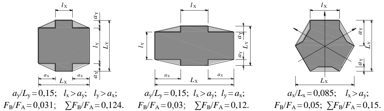
Рисунок 3.4 (продолжение) – Примеры регулярных в плане зданий
