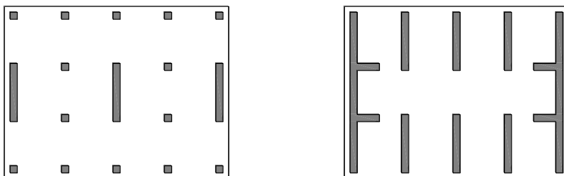
Рисунок 2.5 – Примеры конструктивных систем с ортогональной ориентацией вертикальных конструктивных элементов в плане, но разной горизонтальной жесткостью и сопротивляемостью сейсмическим воздействиям в главных ортогональных направлениях
