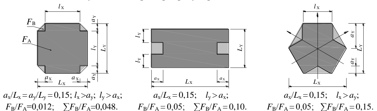
Рисунок 3.4 – Примеры регулярных в плане зданий
