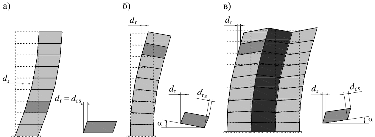
7.2-суреті – Қабаттардың қисаюын анықтау үшін
