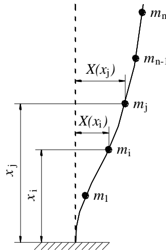
Рисунок 6.2 – К определению значений коэффициентов \eta_{ik}
