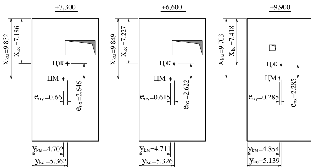
В.3-сурет – Қабатаралық арақабырғалардың деңгейіндегі масса және қаттылық орталықтарының жағдайы
