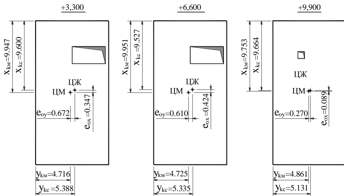
В.5-сурет – Қабатаралық арақабырғалардың деңгейіндегі масса және қаттылық орталықтарының жағдайы
