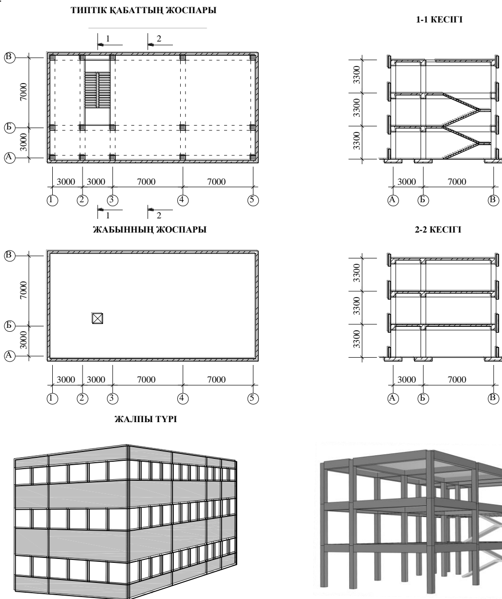
В.1-сурет – Ғимарат пен қаңқаның схемалық жоспары, кесігі және жалпы түрі
